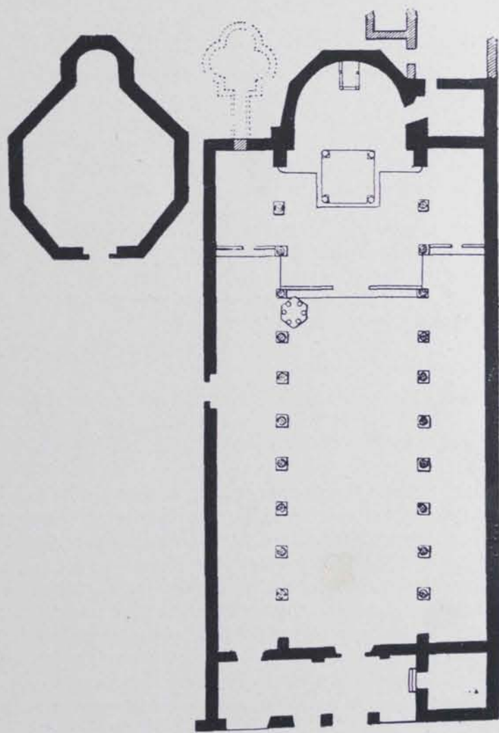
Fig. 220. — Basílica de Grado. Escala 1:400
